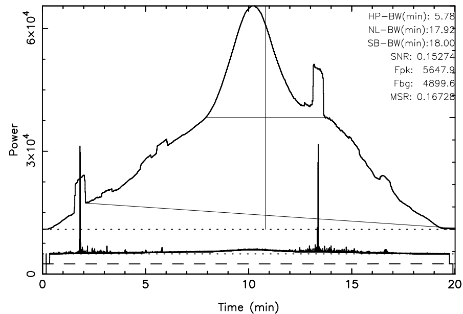
FUJI 3C392 2024/09/05(249)19:37:43-19:57:44JST
