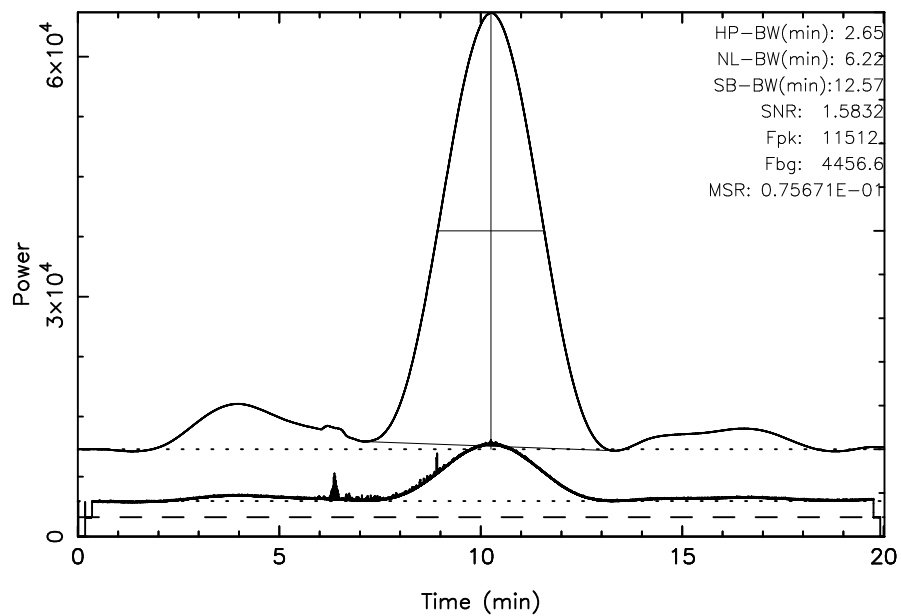
FUJI 3C405 2024/09/05(249)20:40:31-21:00:32JST
