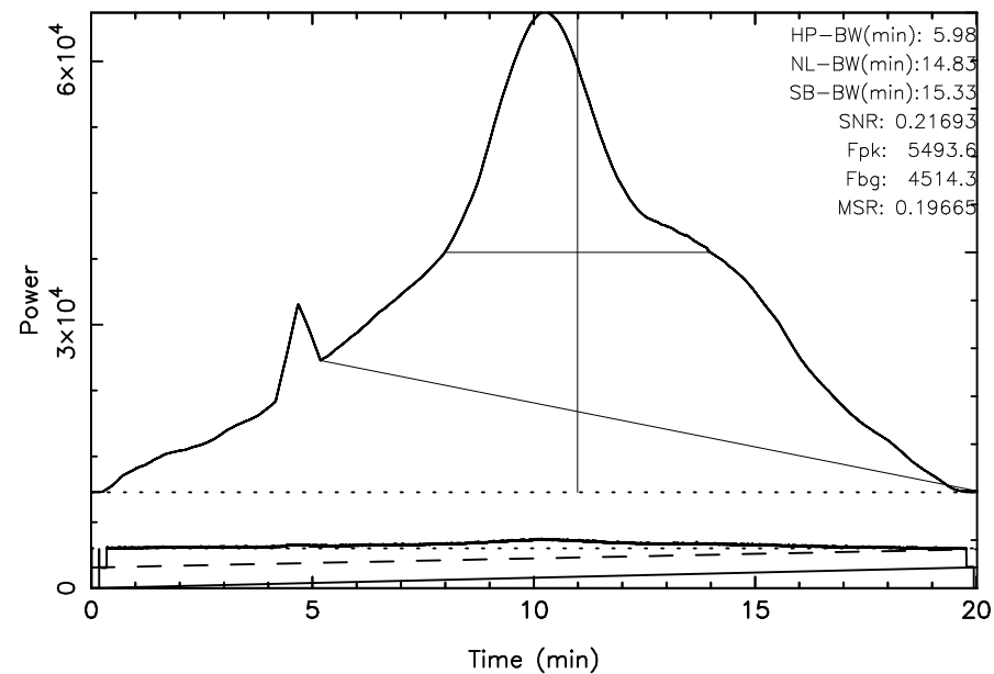
FUJI 3C392 2024/09/14(258)19:02:19-19:22:20JST
