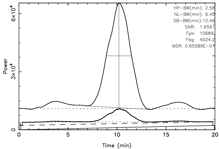
FUJI 3C405 2024/09/14(258)20:05:08-20:25:08JST
