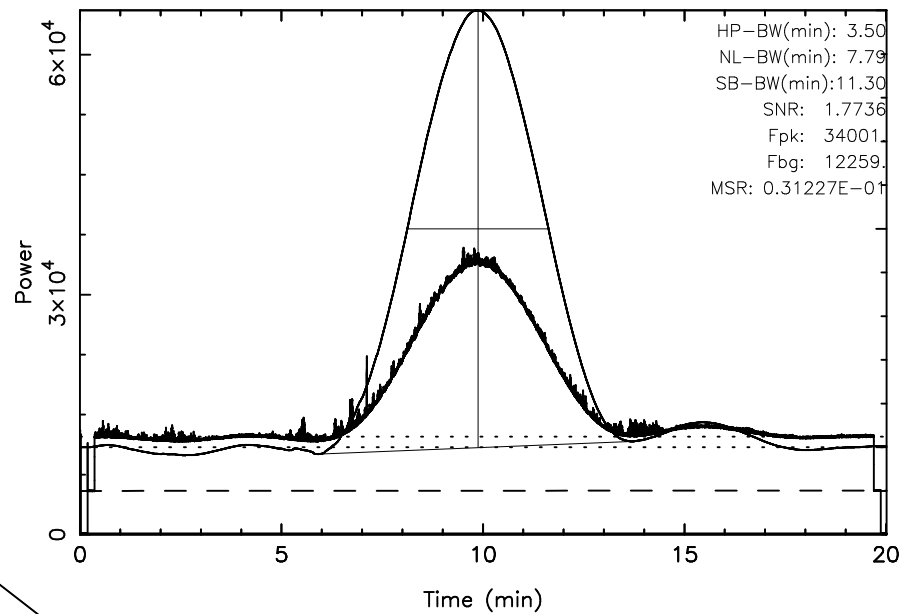
KISO 3C405 2024/09/25(269)19:21:53-19:41:54JST
