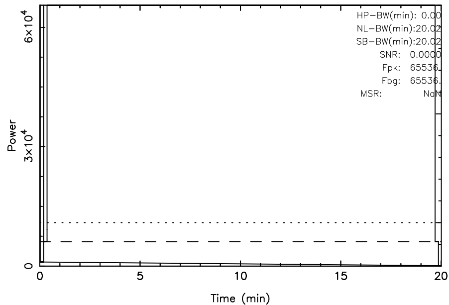
KISO 3C144 2024/09/25(269)04:59:55-05:19:56JST
