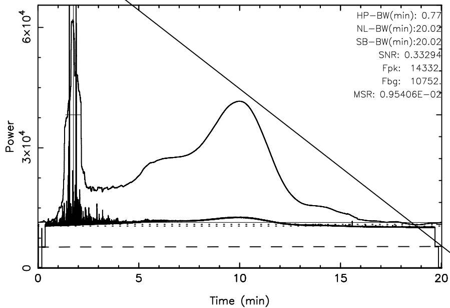
KISO 3C392 2024/09/25(269)18:19:05-18:39:06JST
