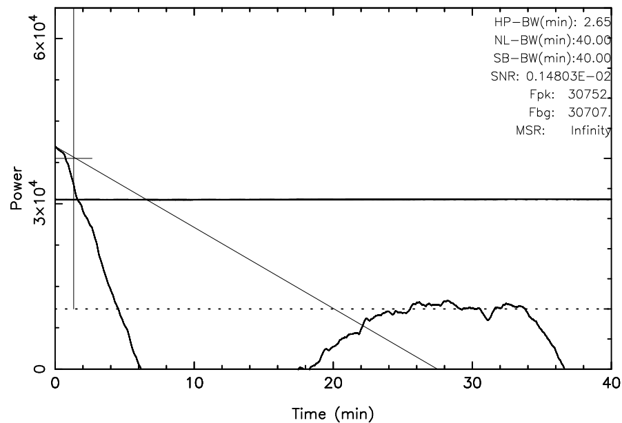
TOYOKAWA 3C10 2024/09/03(247)01:08:05-01:48:05JST
