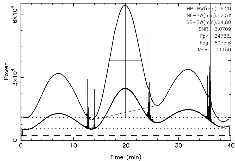
TOYOKAWA 3C405 2024/09/03(247)20:38:24-21:18:24JST
