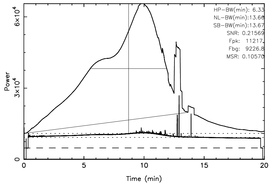
KISO 3C392 2024/10/05(279)17:39:45-17:59:46JST
