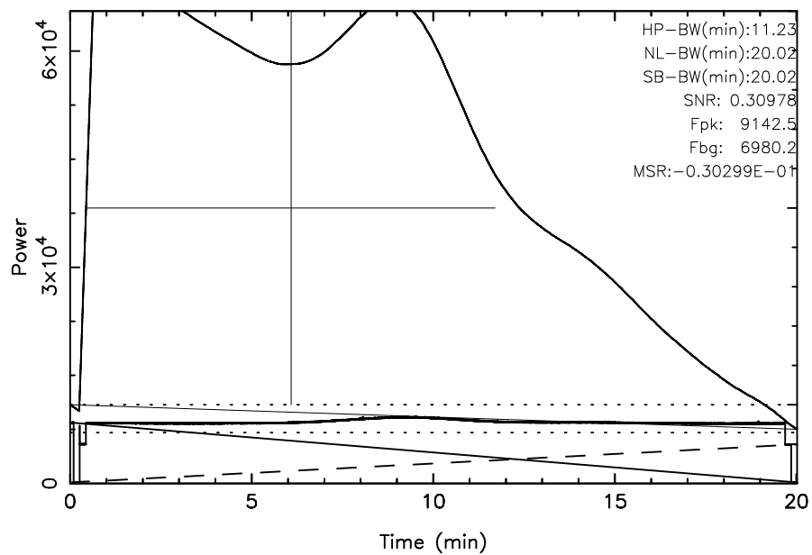
KISO 3C157 2024/10/07(281)04:56:09-05:16:10JST
