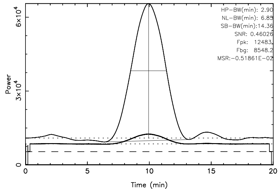
KISO 3C144 2024/10/07(281)04:12:44-04:32:45JST
