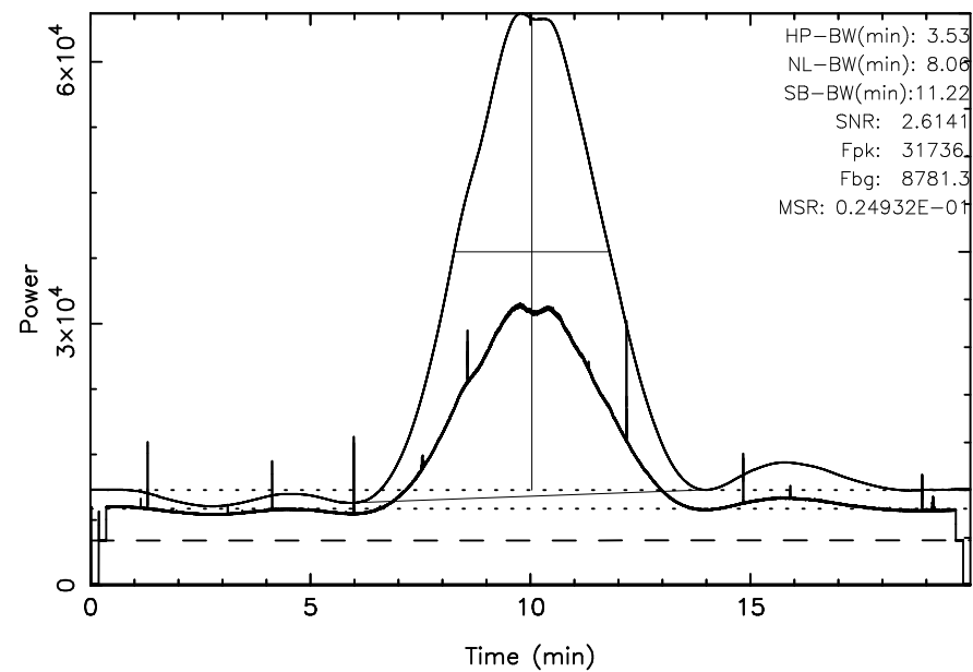
KISO 3C405 2024/10/07(281)18:34:43-18:54:43JST
