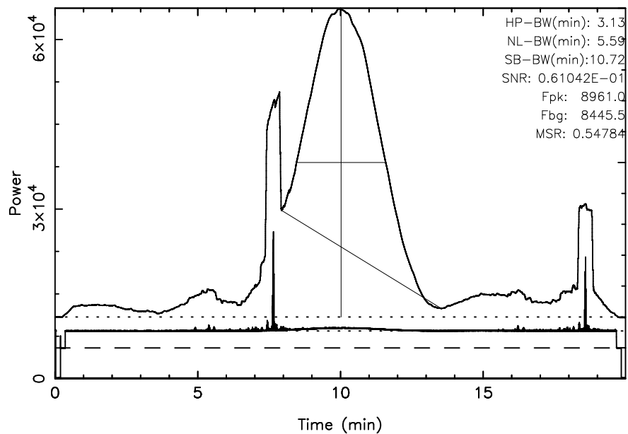
KISO 3C123 2024/10/07(281)03:15:33-03:35:32JST
