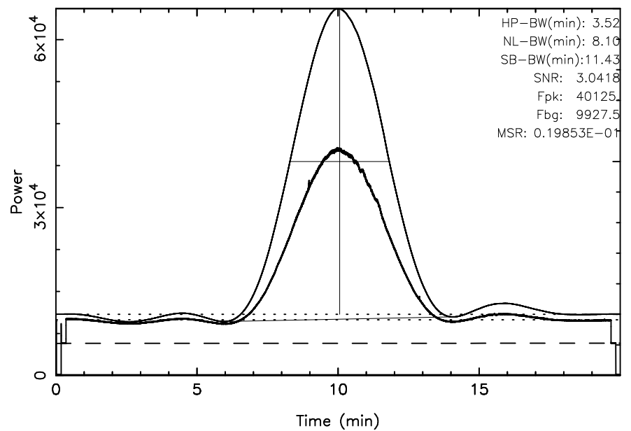
KISO 3C405 2024/10/08(282)18:30:47-18:50:47JST
