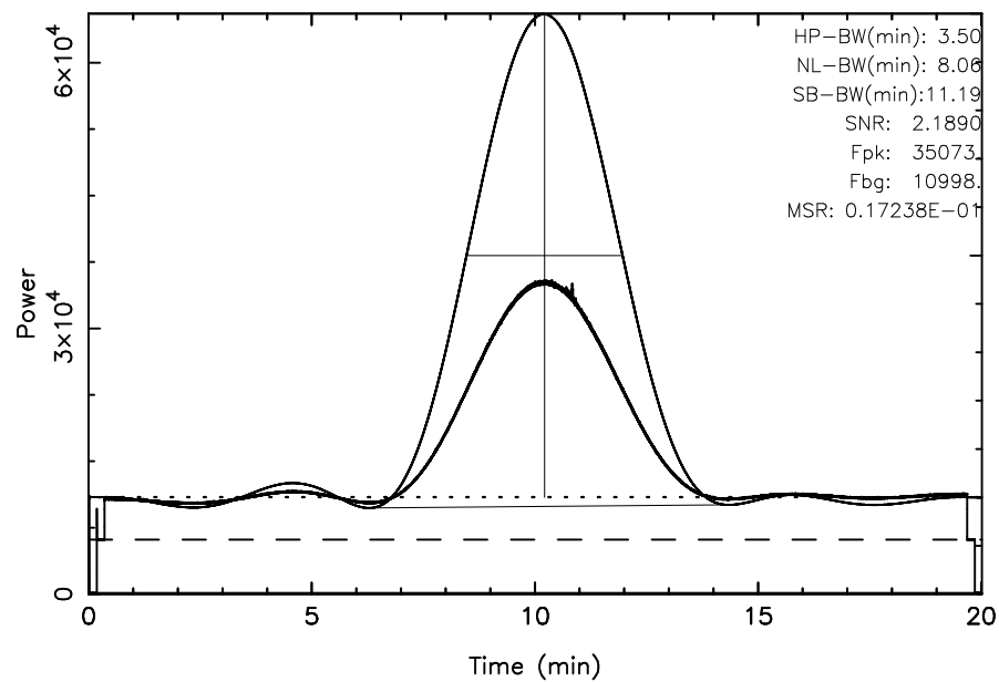
KISO 3C405 2024/10/10(284)18:22:54-18:42:55JST
