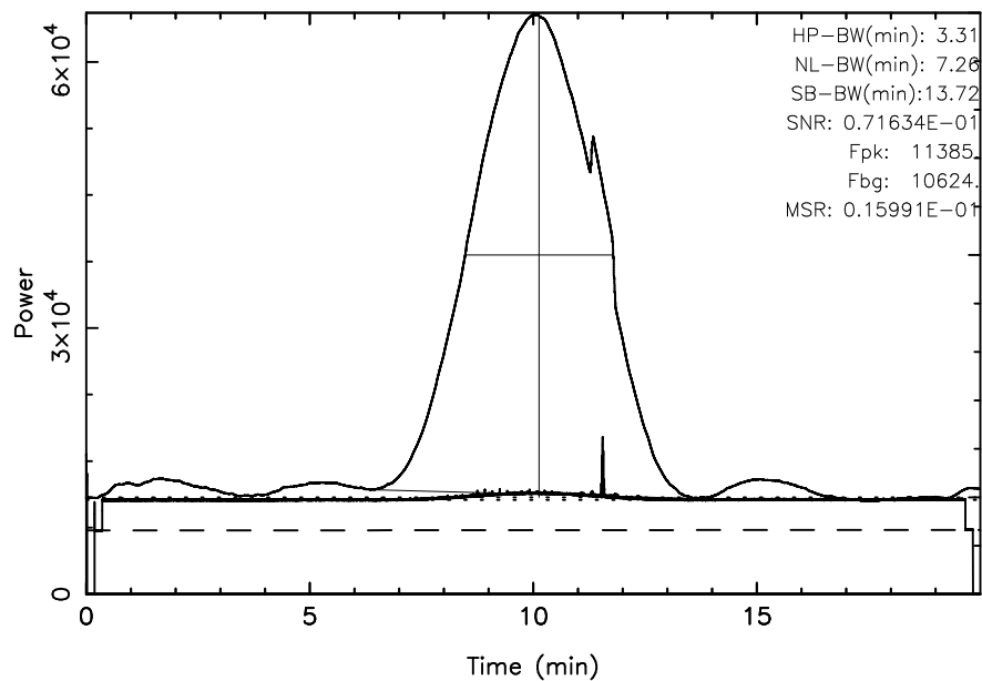
KISO 3C123 2024/10/10(284)03:03:45-03:23:45JST
