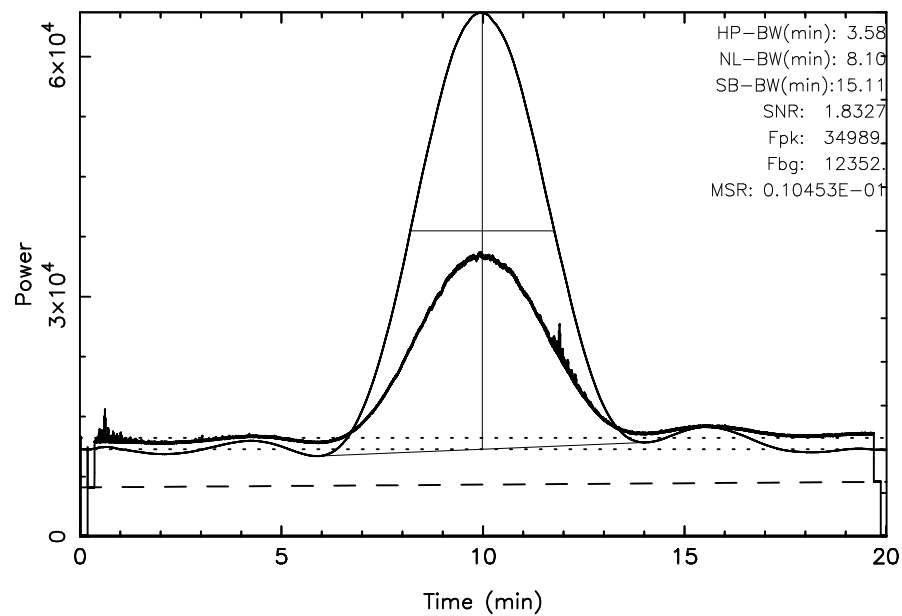
KISO 3C405 2024/10/11(285)18:18:58-18:38:59JST
