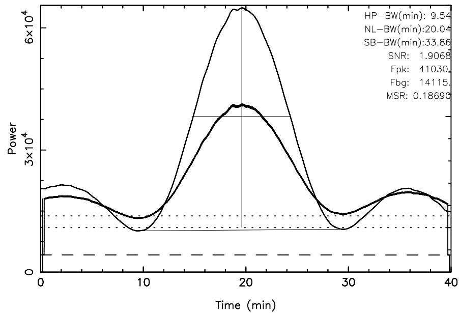
TOYOKAWA 3C461 2024/10/02(276)22:07:59-22:47:59JST
