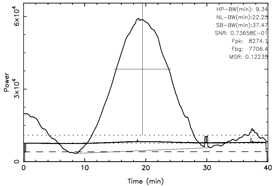
TOYOKAWA 3C10 2024/10/02(276)23:10:07-23:50:07JST
