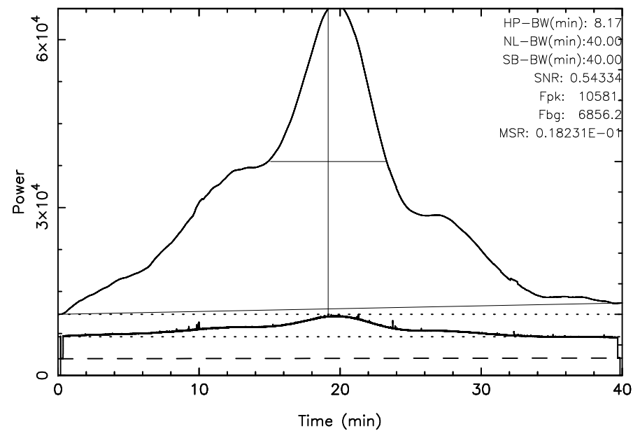
TOYOKAWA 3C392 2024/10/05(279)17:29:46-18:09:46JST
