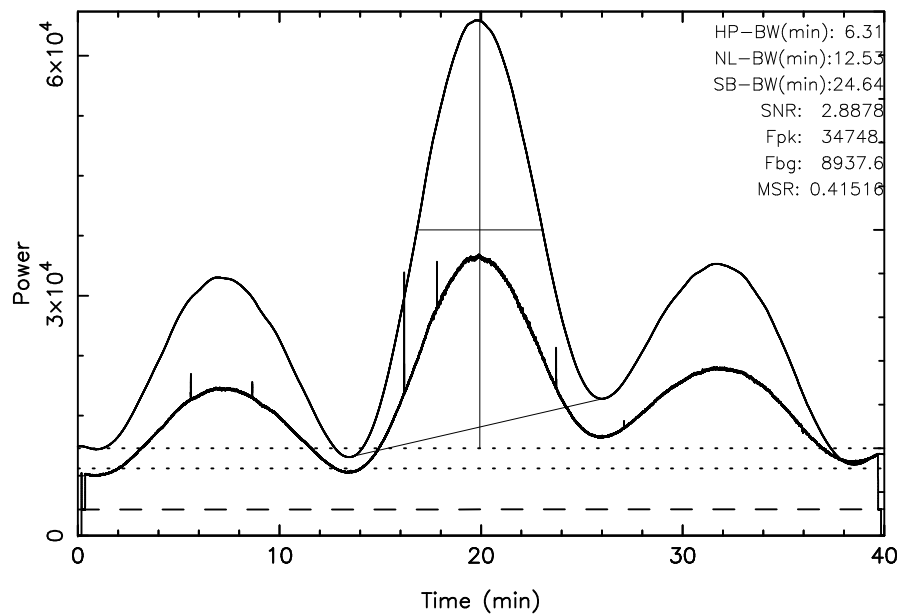
TOYOKAWA 3C405 2024/10/05(279)18:32:35-19:12:35JST
