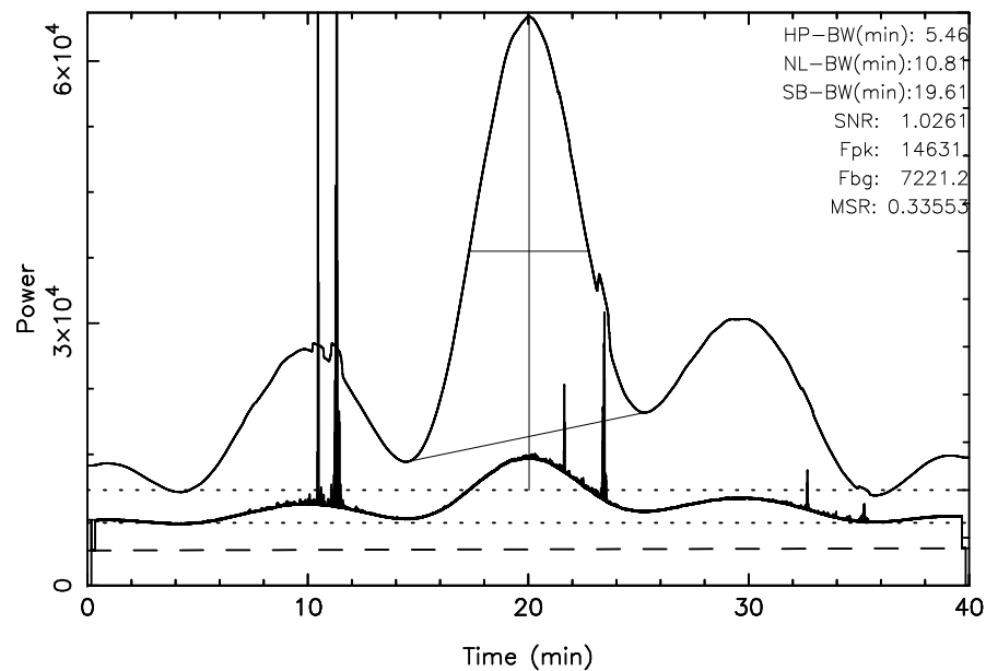
TOYOKAWA 3C144 2024/10/22(296)03:03:47-03:43:47JST
