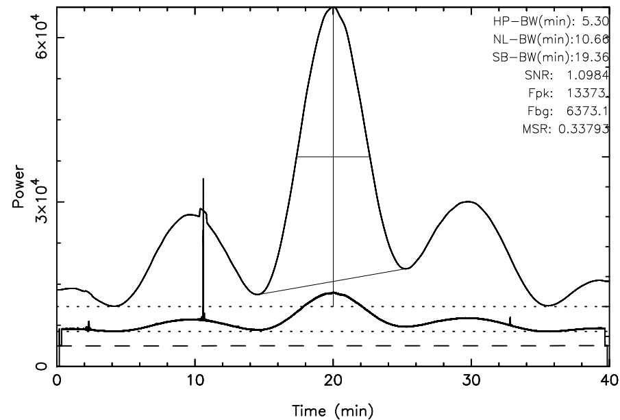
TOYOKAWA 3C144 2024/10/24(298)02:55:55-03:35:55JST
