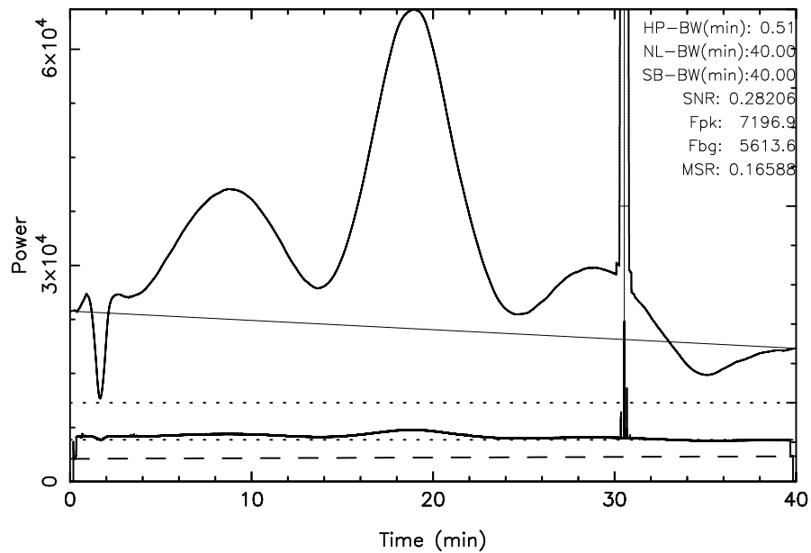
TOYOKAWA 3C157 2024/10/24(298)03:39:19-04:19:19JST
