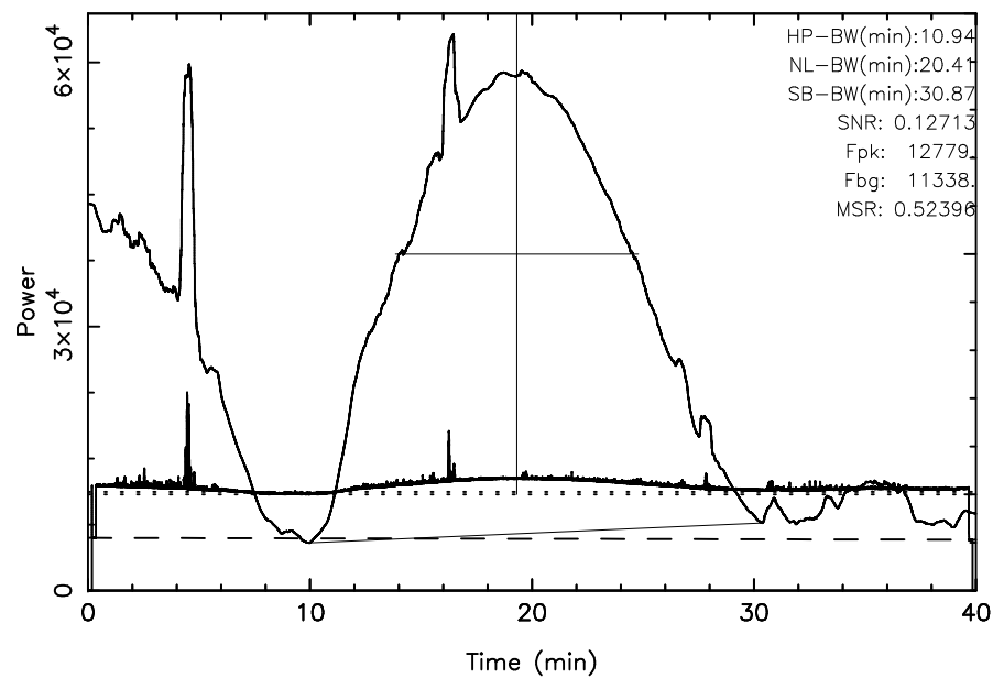
TOYOKAWA 3C10 2024/11/27(332)19:29:57-20:09:57JST
