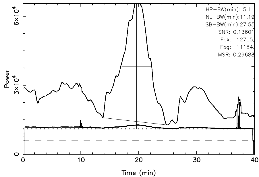
TOYOKAWA 3C157 2025/01/08(008)22:36:35-23:16:35JST
