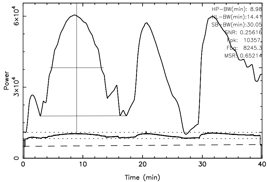
TOYOKAWA 3C123 2025/02/08(039)18:54:05-19:34:05JST
