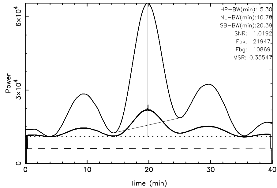
TOYOKAWA 3C144 2025/02/08(039)19:51:18-20:31:18JST
