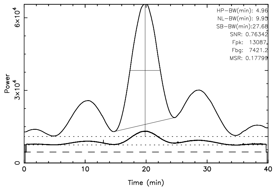
TOYOKAWA 3C274 2025/04/12(102)22:38:32-23:18:32JST
