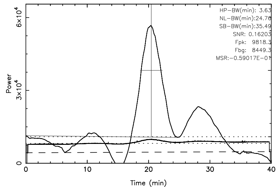
TOYOKAWA 3C348 2025/04/15(105)02:50:15-03:30:15JST
