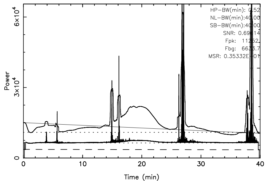
TOYOKAWA 3C348 2025/04/27(117)02:03:04–02:43:04JST
