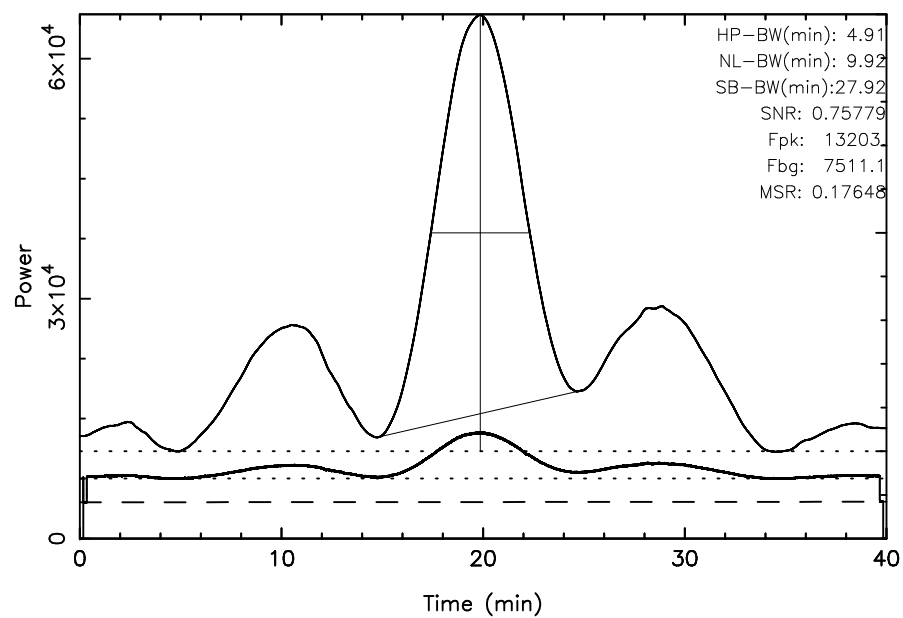
TOYOKAWA 3C274 2025/04/29(119)21:31:41-22:11:41JST
