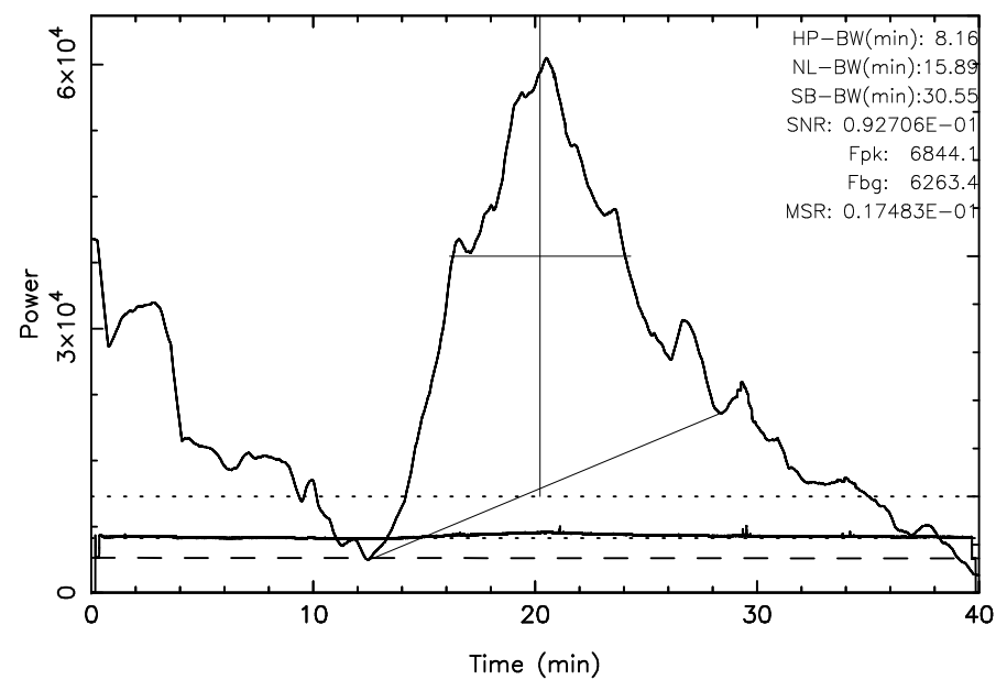
TOYOKAWA 3C295 2025/04/29(119)23:11:33-23:51:33JST
