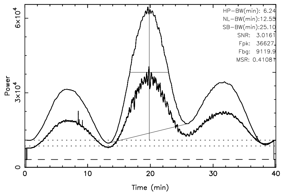
TOYOKAWA 3C405 2025/05/24(144)03:24:21-04:04:21JST
