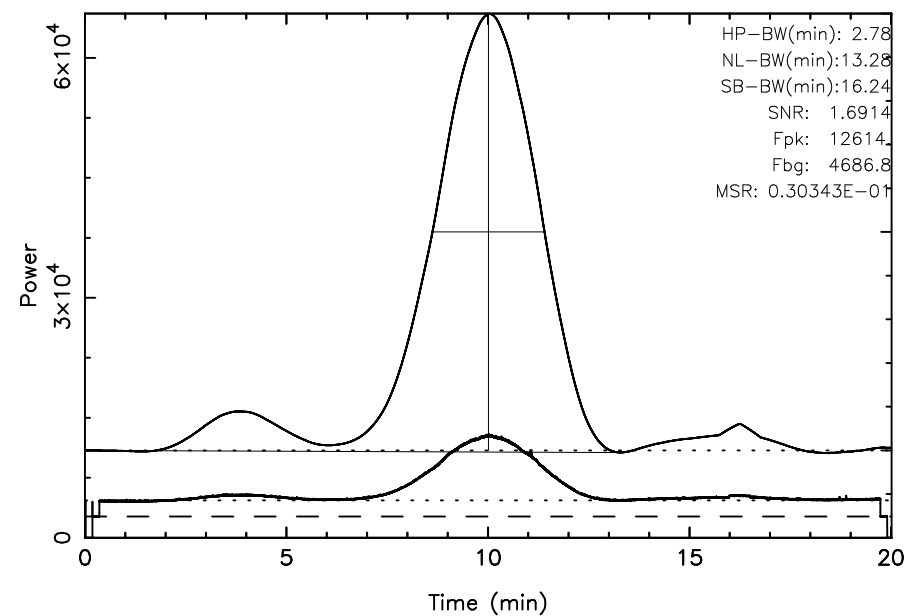
FUJI 3C405 2025/06/27(178)01:20:39-01:40:40JST
