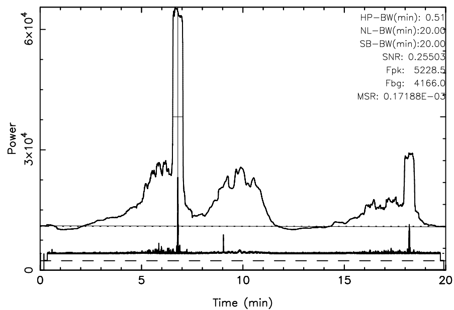
FUJI 3C348 2025/06/27(178)22:09:17-22:29:17JST
