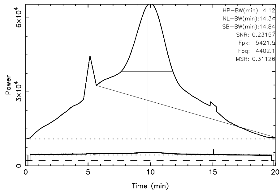
FUJI 3C392 2025/07/23(204)22:31:42–22:51:42JST
