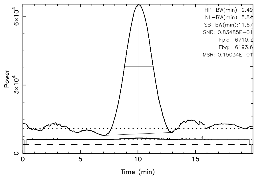
KISO 3C348 2025/07/23(204)20:27:05–20:47:05JST
