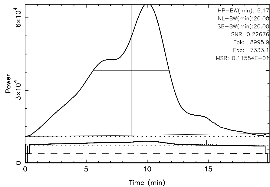
KISO 3C392 2025/07/23(204)22:31:42–22:51:42JST
