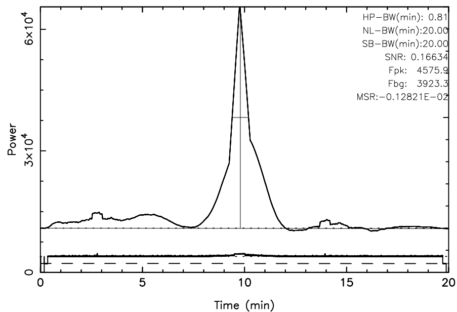
FUJI 3C348 2025/07/23(204)20:27:05–20:47:05JST
