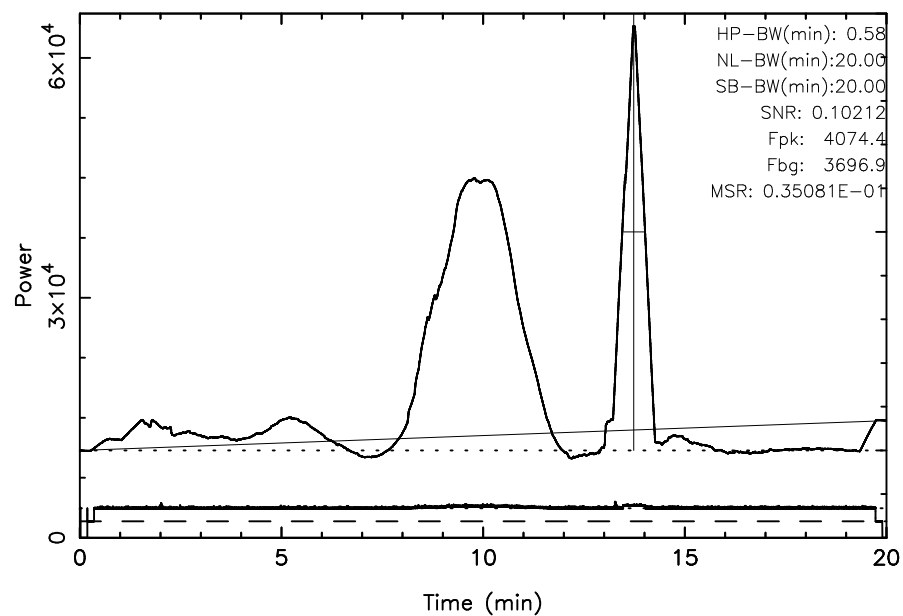
FUJI 3C348 2025/07/24(205)20:23:09–20:43:09JST
