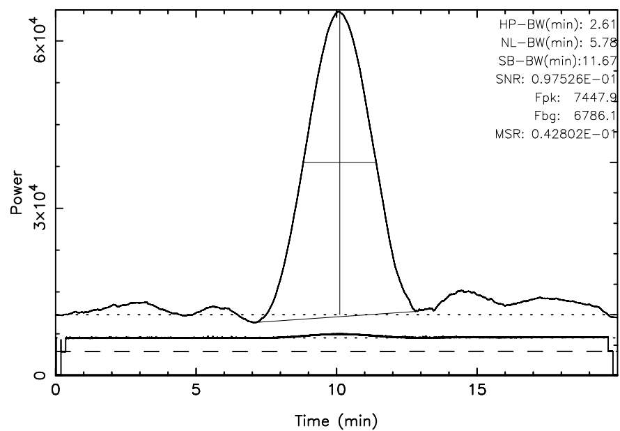
KISO 3C348 2025/07/24(205)20:23:09–20:43:09JST
