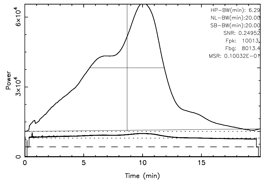
KISO 3C392 2025/07/24(205)22:27:46–22:47:46JST
