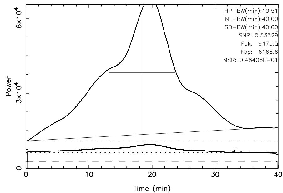
TOYOKAWA 3C392 2025/07/24(205)22:17:47–22:57:47JST
