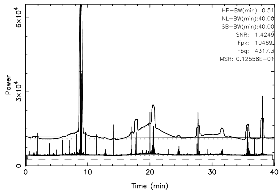
TOYOKAWA 3C123 2025/09/12(255)04:44:51-05:24:51JST
