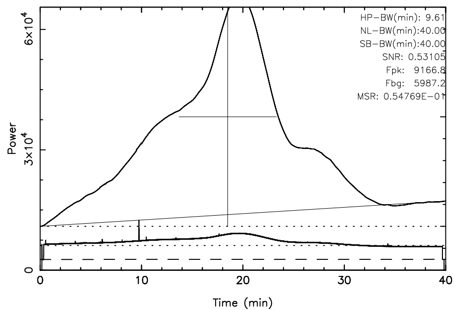
TOYOKAWA 3C392 2025/09/12(255)19:01:12-19:41:12JST
