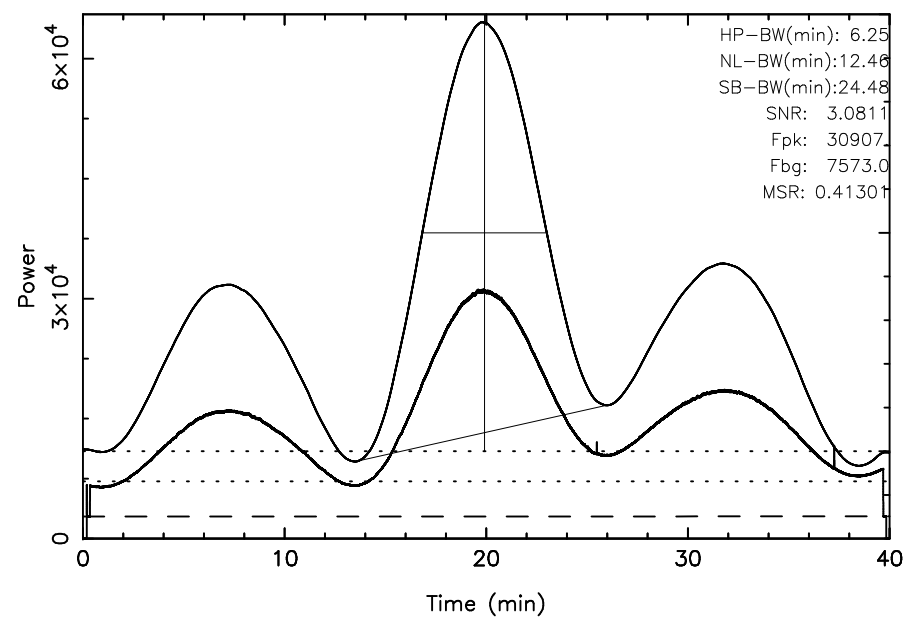
TOYOKAWA 3C405 2025/09/12(255)20:04:00-20:44:00JST
