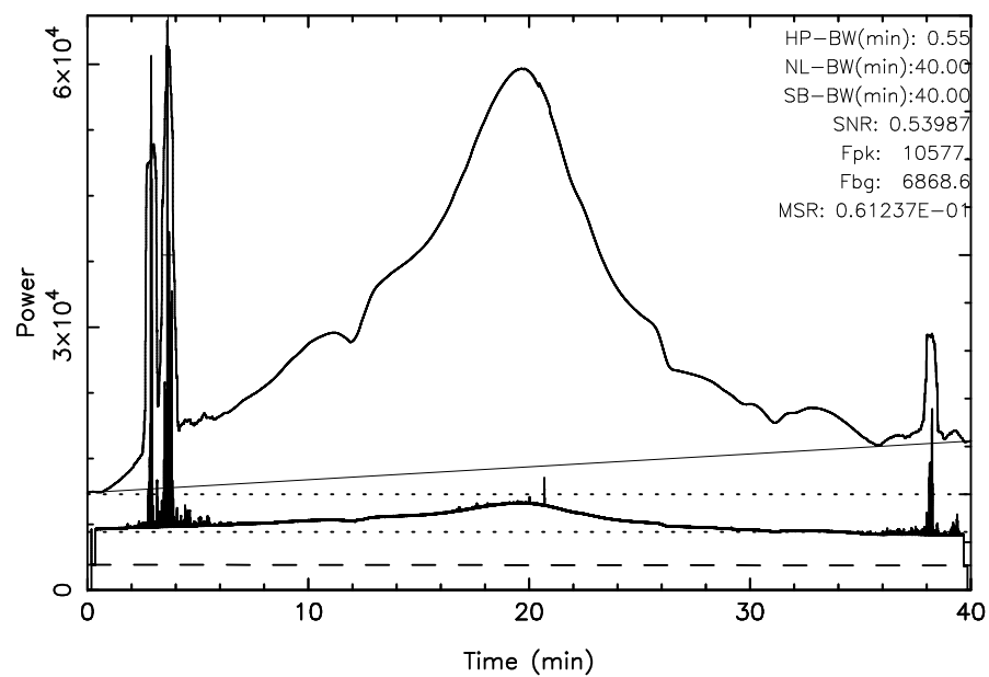
TOYOKAWA 3C392 2025/09/22(265)18:21:53-19:01:53JST
