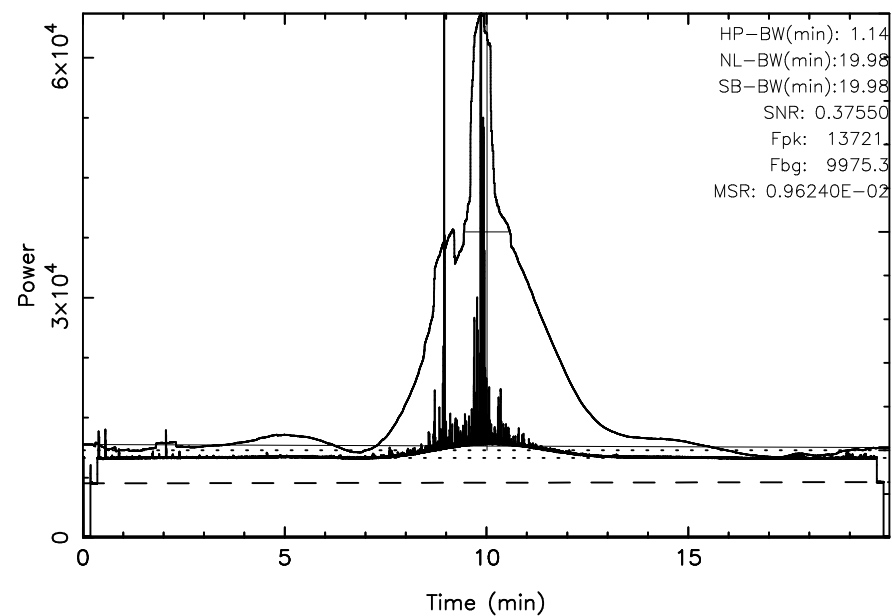
KISO 3C144 2025/10/15(288)03:42:19–04:02:18JST
