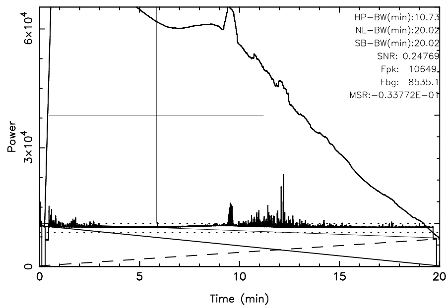
KISO 3C157 2025/10/15(288)04:25:42–04:45:43JST
