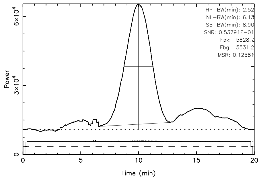
FUJI 3C123 2025/10/15(288)02:45:05-03:05:05JST
