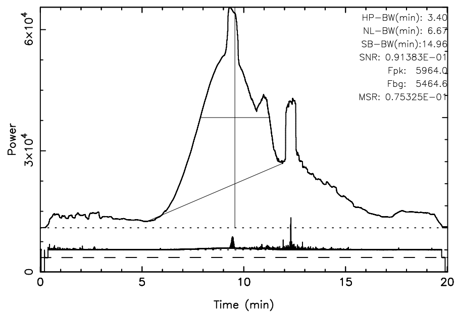
FUJI 3C157 2025/10/15(288)04:25:42-04:45:43JST
