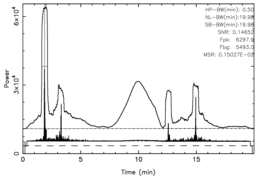
FUJI 3C123 2025/10/20(293)02:25:27-02:45:26JST
