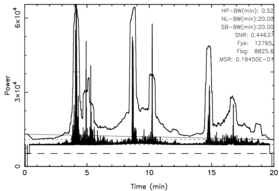
FUJI 3C157 2025/10/24(297)03:50:20-04:10:20JST
