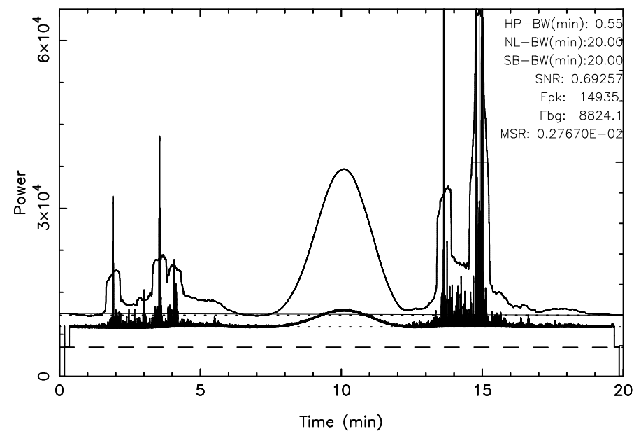
FUJI 3C144 2025/10/24(297)03:06:55-03:26:55JST
