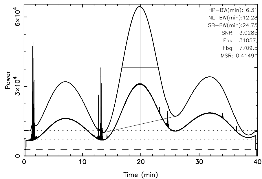
TOYOKAWA 3C405 2025/10/16(289)17:50:19–18:30:19JST
