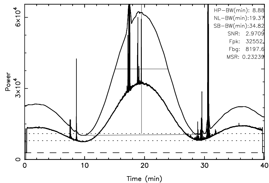
TOYOKAWA 3C461 2025/10/26(299)20:34:37-21:14:37JST
