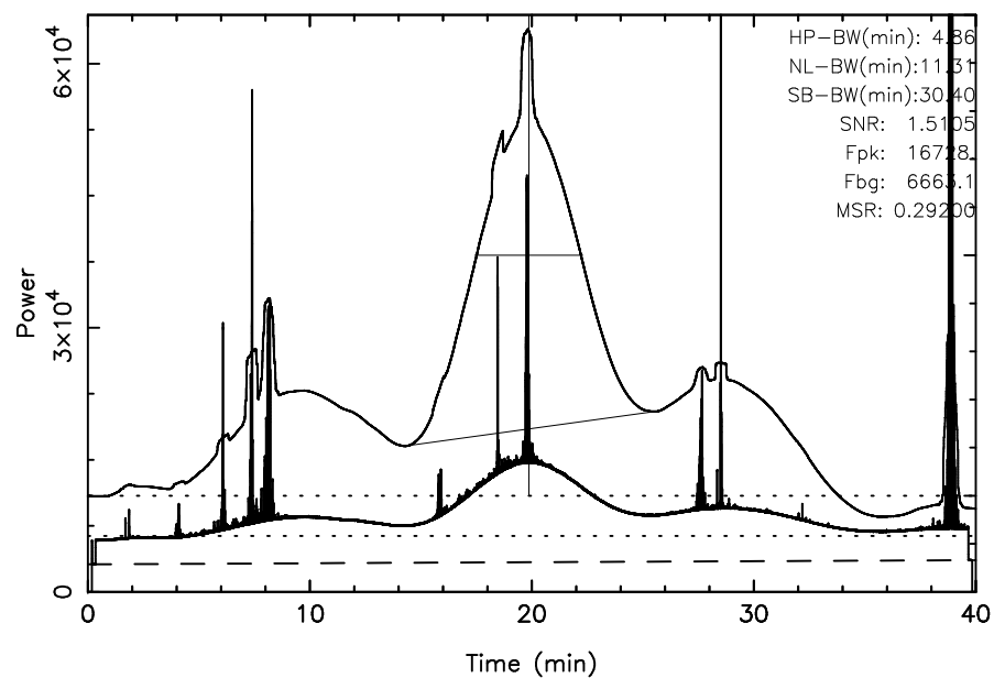
TOYOKAWA 3C144 2025/11/29(333)00:35:23-01:15:23JST
