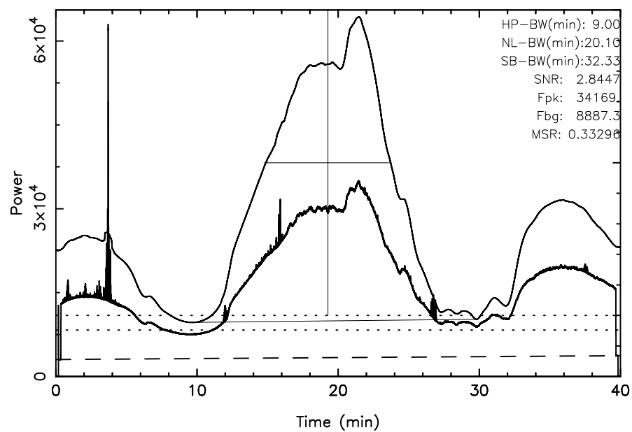
TOYOKAWA 3C461 2025/11/29(333)18:20:57-19:00:57JST
