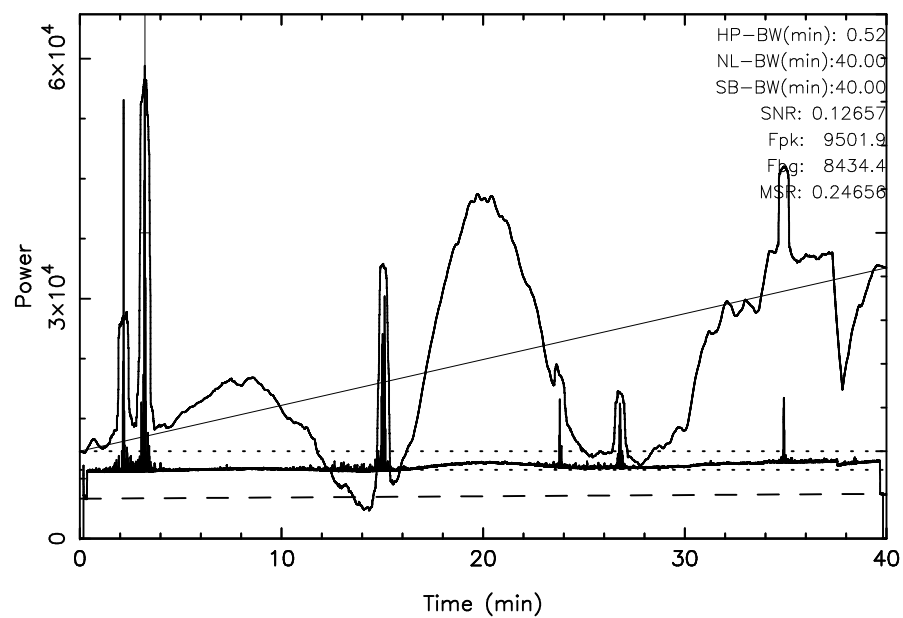
TOYOKAWA 3C123 2026/01/29(029)19:34:25-20:14:25JST
