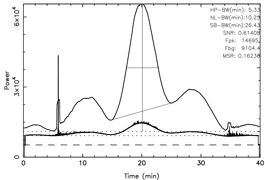
TOYOKAWA 3C274 2026/02/07(038)02:55:05-03:35:05JST
